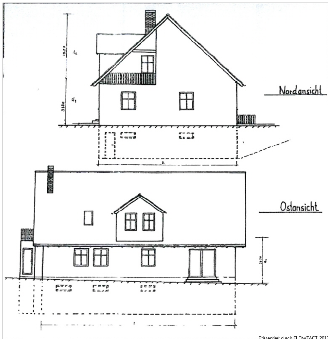
Ansichten 2
